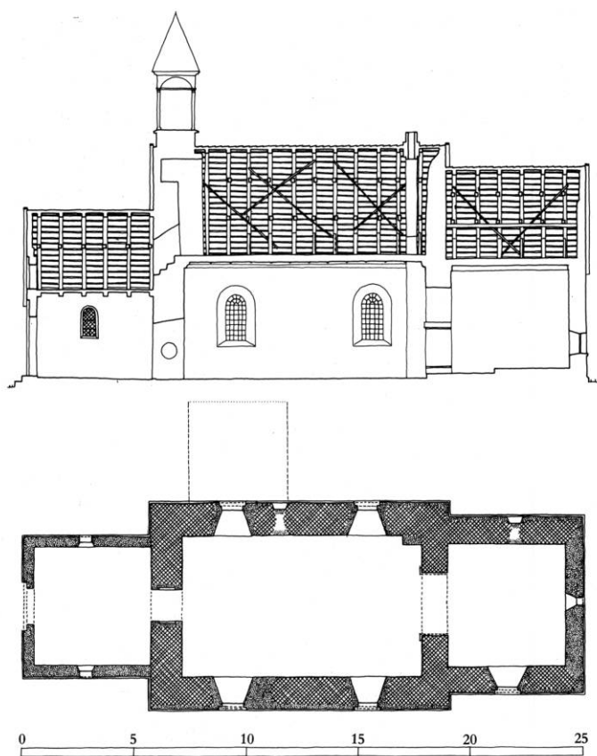
Fig. 8. Længdesnit og grundplan 1:300. Tegnet af KdeFL efter skitseopmåling 1963 ved Strange Nielsens tegnestue, Skanderborg. På grundplanen er angivet placering og en mulig længde af forsvundet våbenhus på skibets nordside (s. 3376 og note 22). - Longitudinal section and ground-plan.
